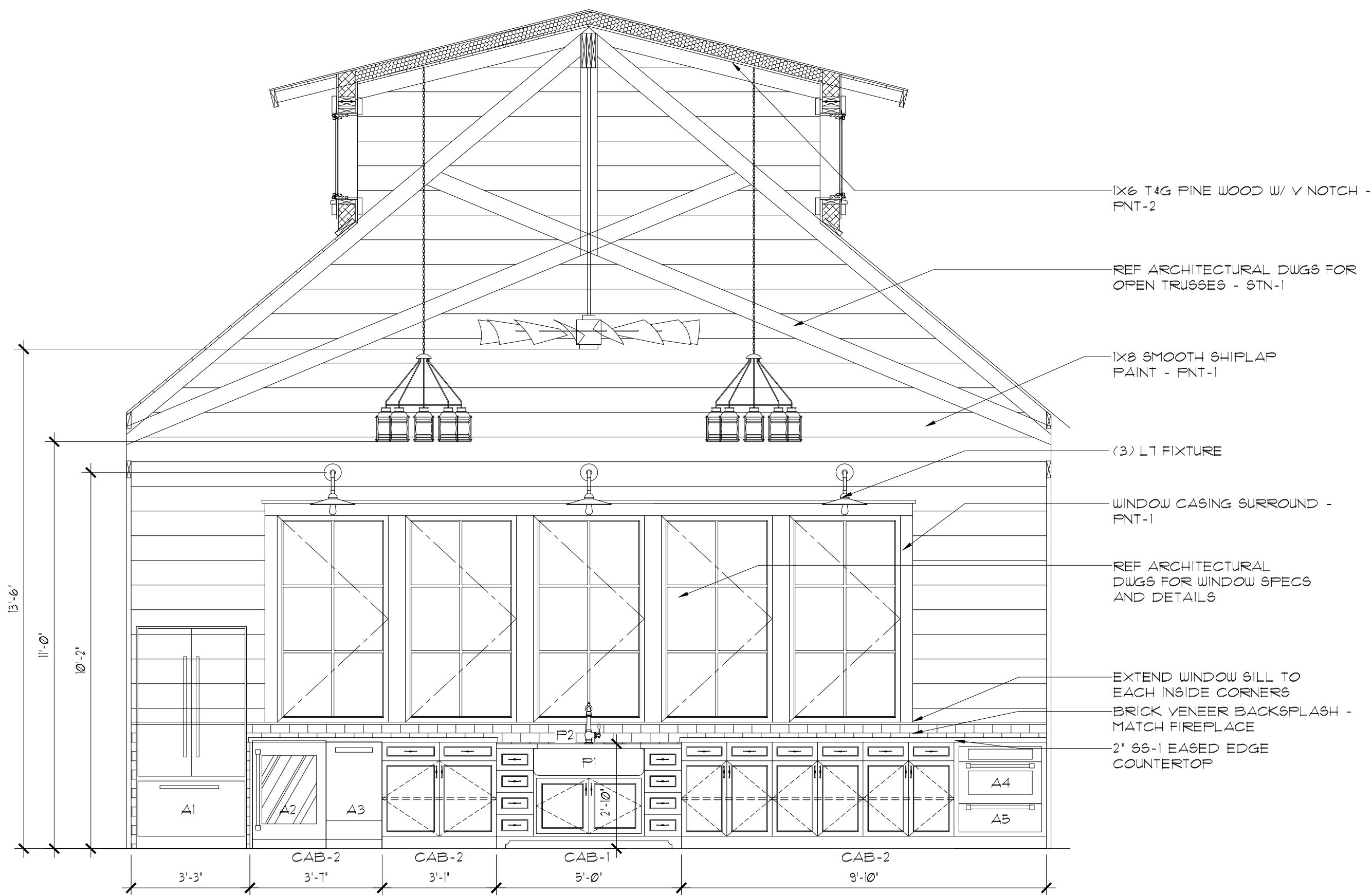
3 RM 102 - WEST WALL SCALE: 3/8" = 1'-0"
