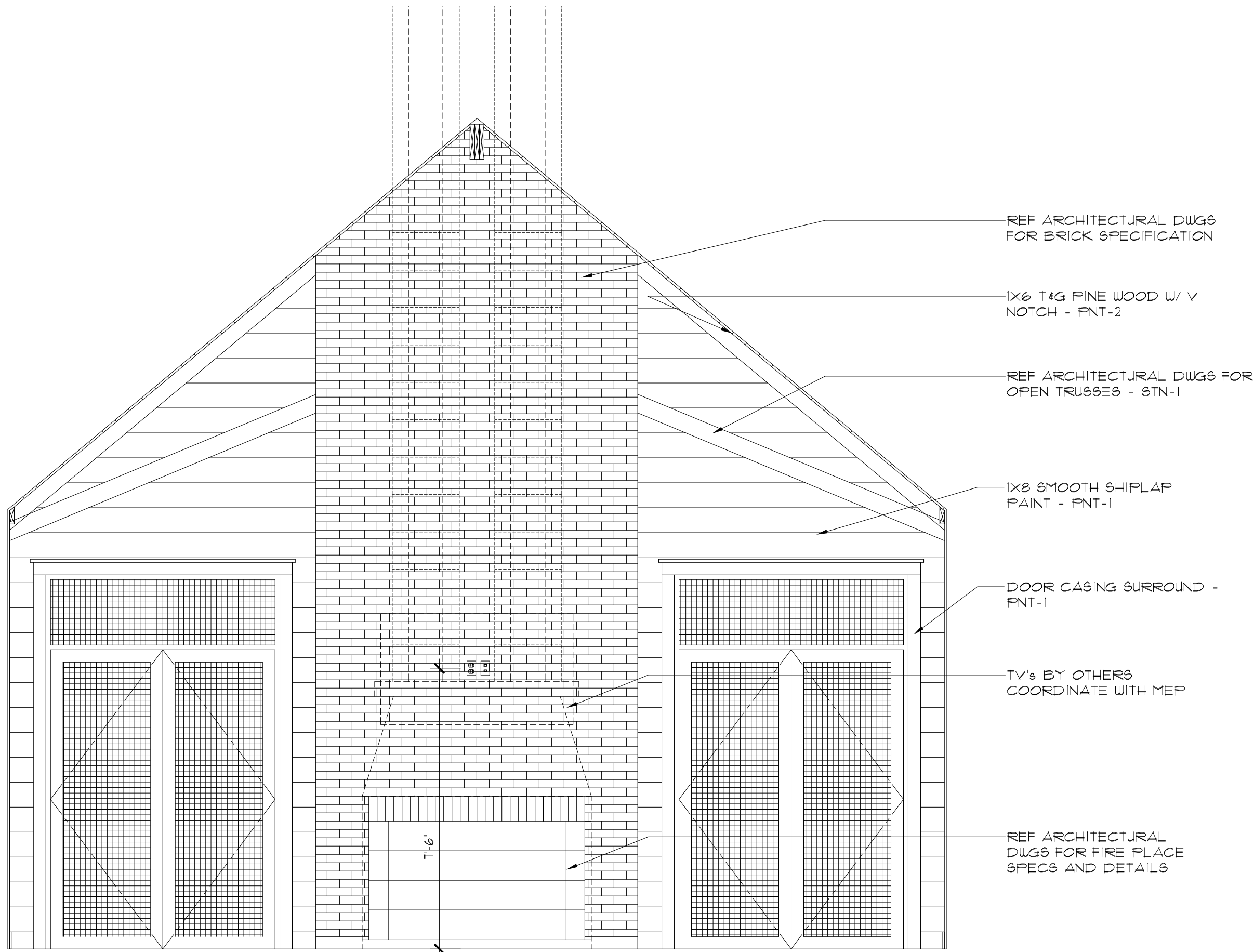
1 RM 103 - NORTH SCALE: 3/8" = 1'-0"
